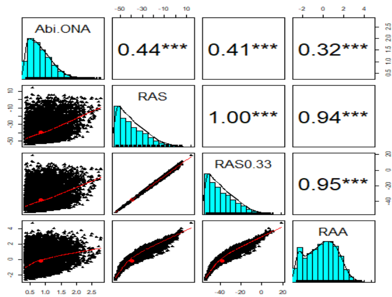
نمودار ۶. همبستگی نمره‌های خطرپذیری با توانایی متداول برای افراد قوی (ریاضی)
