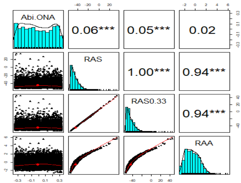
نمودار ۵. همبستگی نمره‌های خطرپذیری با توانایی متداول برای افراد متوسط (ریاضی)
