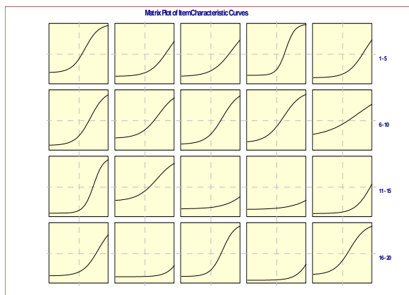
نمودار ۶. منحنی‌های ویژگی تمامی سؤالات آزمون درس فلسفه در مدل سه پارامتری
