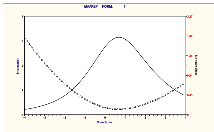
نمودار ۳. منحنی آگاهی و منحنی خطای استاندارد آزمون درس روان‌شناسی
