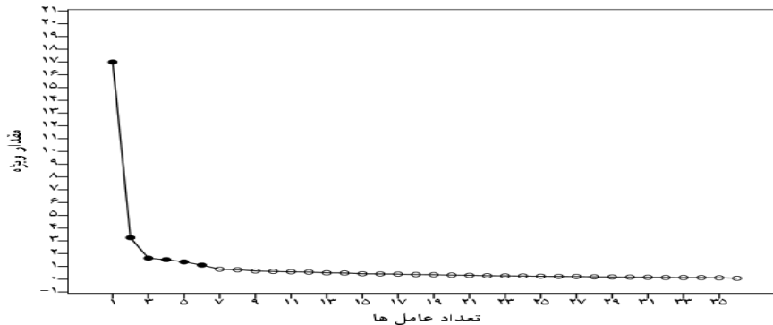
شکل ۱. نمودار سنگ‌ریزه جهت تعیین تعداد عوامل مکنون
